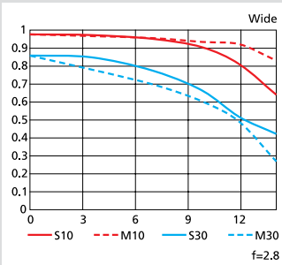
MTF-käyrät
